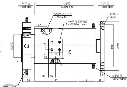
MAPH200W-03 尺寸图
