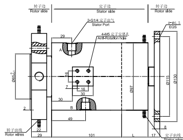
MAPH200W-03 尺寸图
